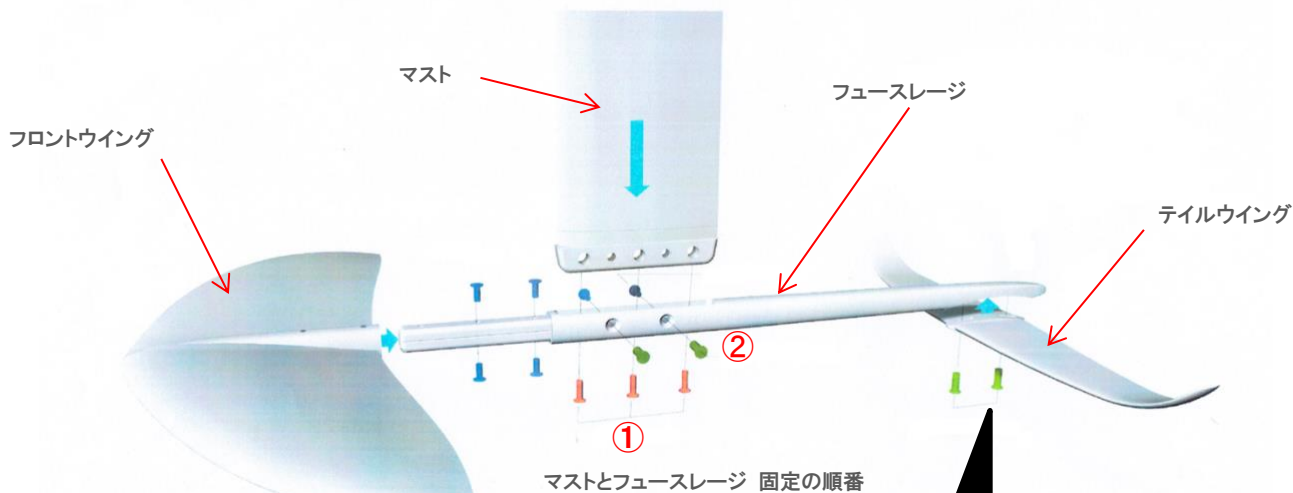
図2. FOIL 各パーツ名称と組み立て方法
